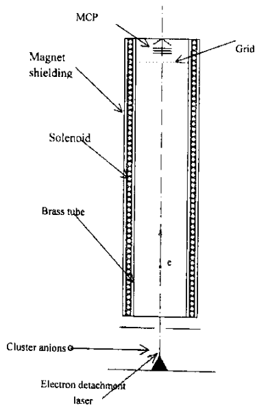
图 2 实验装置中光电子能谱仪详细结构
