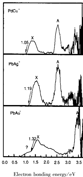
图 4 实验得到的 \text{PbCu}^- 、 \text{PbAg}^- 和 \text{PbAu}^- 的光电子能谱图
