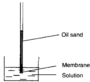
图 1 测定接触角的简明示意图
