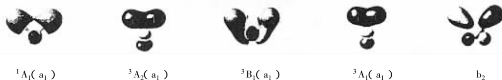
图 1 分子轨道电子云等值面图
