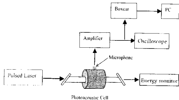
图1 光声实验装置简图
