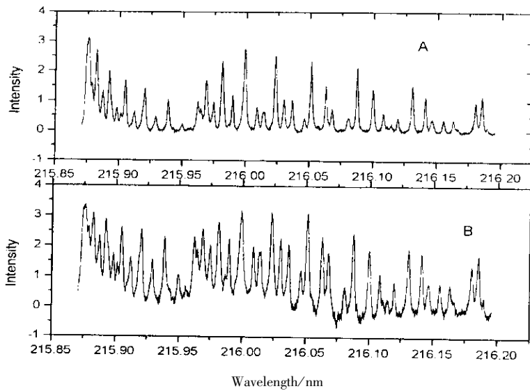
图4 C_2H_2 第一电子激发态 A^1A_uV^4K^1 振动态的脉冲光声光谱 A 和 LIF 谱 B
