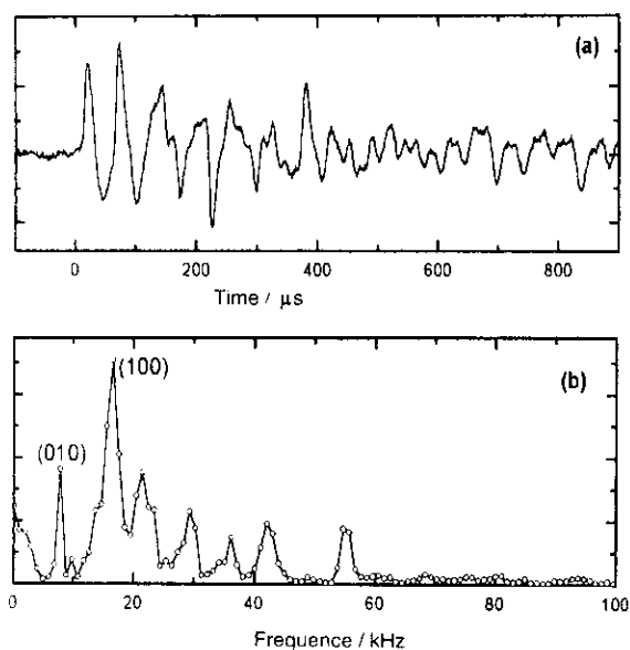
图 2 脉冲光声信号
