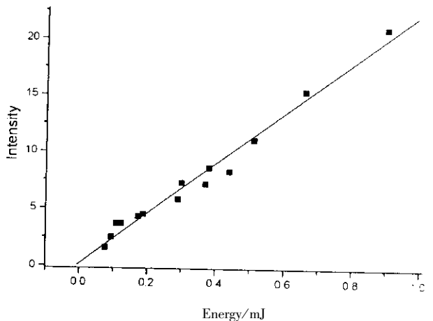
图6 光声信号与激光能量的关系
