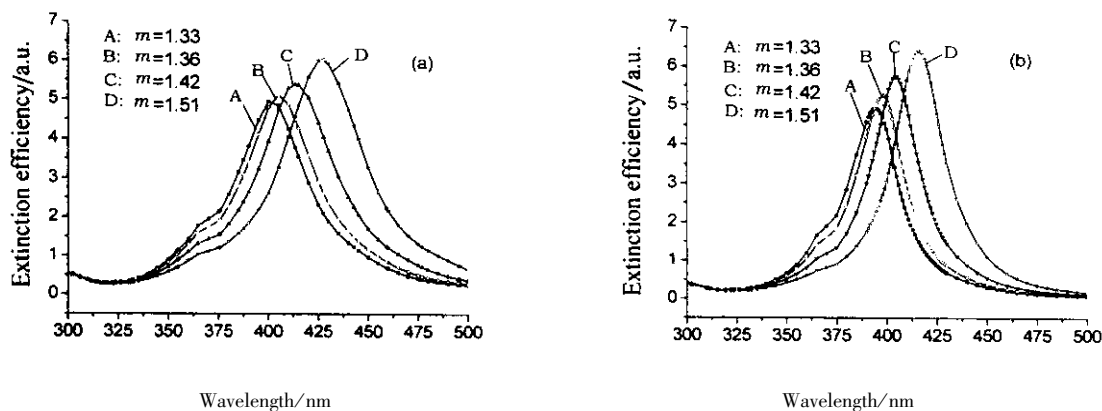
图 2 不同介电环境中的球状银纳米粒子消光效率的理论计算 (a) 离散偶极近似 (DDA) 的数值计算结果; (b) 米氏方法对相同粒子的计算结果.
